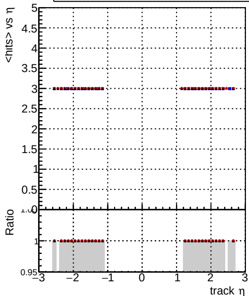
mean hits — DQMstep3_SoftQCD_CKF — DQMstep3_SoftQCD_default — DQMstep3_SoftQCD_defaultNEWT3
