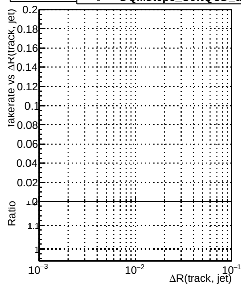
—●— DQMstep3_SoftQCD_CKF —●— DQMstep3_SoftQCD_default —●— DQMstep3_SoftQCD_defaultNEWT3
