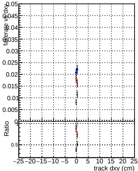
— DOMstep3 SoftOCB-CKF — DOMstep3 SoftOCB-default — DOMstep3 SoftOCB-defaultNEWT3
