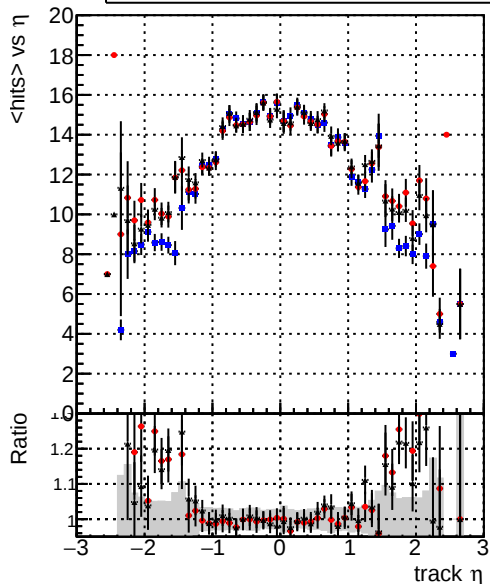
DQMstep3_SoftQCD_CKF DQMstep3_SoftQCD_default DQMstep3_SoftQCD_defaultNEWT3 mean hits
