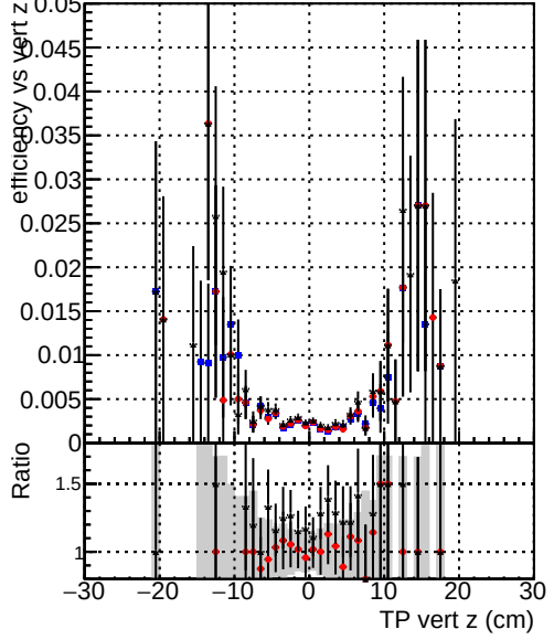
Efficiency vs TP vert z (cm) Legend: DQMstep3_SoftQCD_CKF (blue circles) DQMstep3_SoftQCD_default (red circles) DQMstep3_SoftQCD_defaultNEWT3 (black circles)
