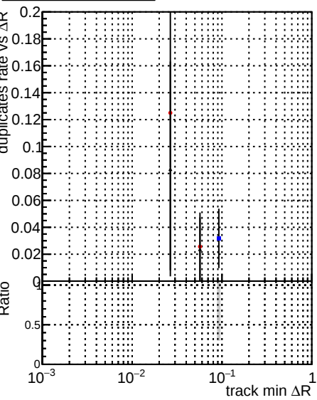
Legend: DQMstep3_SoftQCD_CKF (blue squares), DQMstep3_SoftQCD_default (red circles), DQMstep3_SoftQCD_defaultNEWT3 (black triangles)
