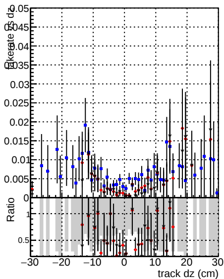
—●— DOMstep3 SoftOCD-CKF —●— DOMstep3 SoftOCD-default —●— DOMstep3 SoftOCD-defaultNEWT3
