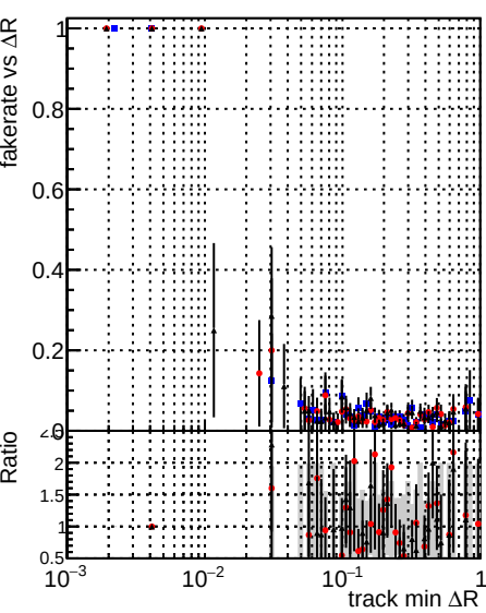
DOMstep3 SoftQCD CKF DOMstep3 SoftQCD default DOMstep3 SoftQCD defaultNEWT3
