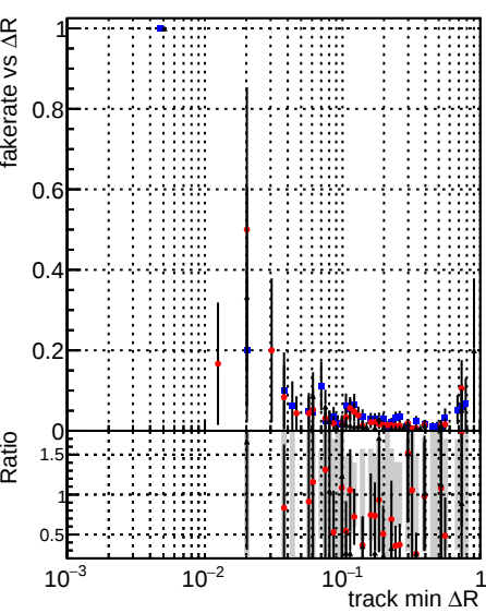
Legend: DQMstep3_SoftQCD_CKF (blue dots), DQMstep3_SoftQCD_default (red dots), DQMstep3_SoftQCD_defaultNEWT3 (grey dots)
