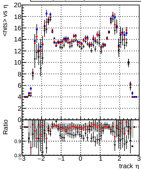
DQMstep3_SoftQCD_CKF DQMstep3_SoftQCD_default DQMstep3_SoftQCD_defaultNEWT3 mean hit
