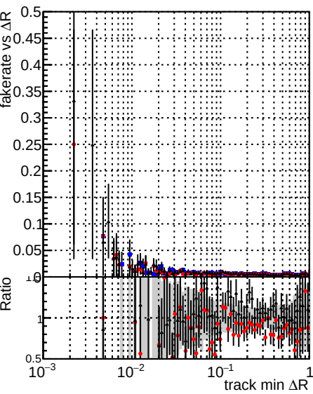
Fake rate vs ΔR(track, jet) DOMstep3_SoftQCD_CKF DOMstep3_SoftQCD_default DOMstep3_SoftQCD_defaultNEWT3
