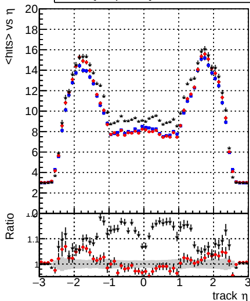
mean hit — DQMstep3_SoftQCD_CKF — DQMstep3_SoftQCD_default — DQMstep3_SoftQCD_defaultNEWT3
