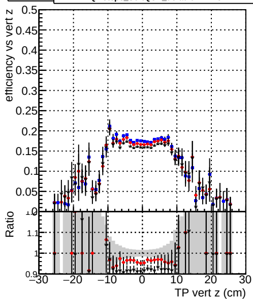
—●— DQMstep3_SoftQCD_CKF —●— DQMstep3_SoftQCD_default —●— DQMstep3_SoftQCD_defaultNEWT3
