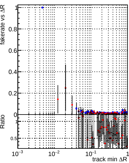
Fake rate vs \Delta R(\text{track, jet}) DQMstep3_SoftQCD_CKF DQMstep3_SoftQCD_default DQMstep3_SoftQCD_defaultNEWT3
