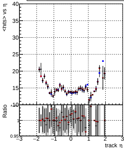
mean hit — DQMstep3_SoftQCD_CKF — DQMstep3_SoftQCD_default — DQMstep3_SoftQCD_defaultNEWT3
