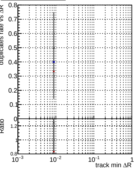
Legend: DQMstep3_SoftQCD_CKF (blue squares), DQMstep3_SoftQCD_default (red circles), DQMstep3_SoftQCD_defaultNEWT3 (black line)
