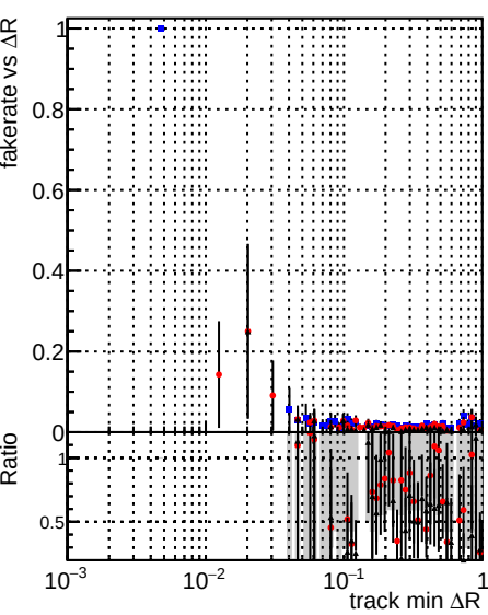
Fake rate vs ΔR(track, jet) Legend: DQMstep3_SoftQCD_CKF DQMstep3_SoftQCD_default DQMstep3_SoftQCD_defaultNEWT3
