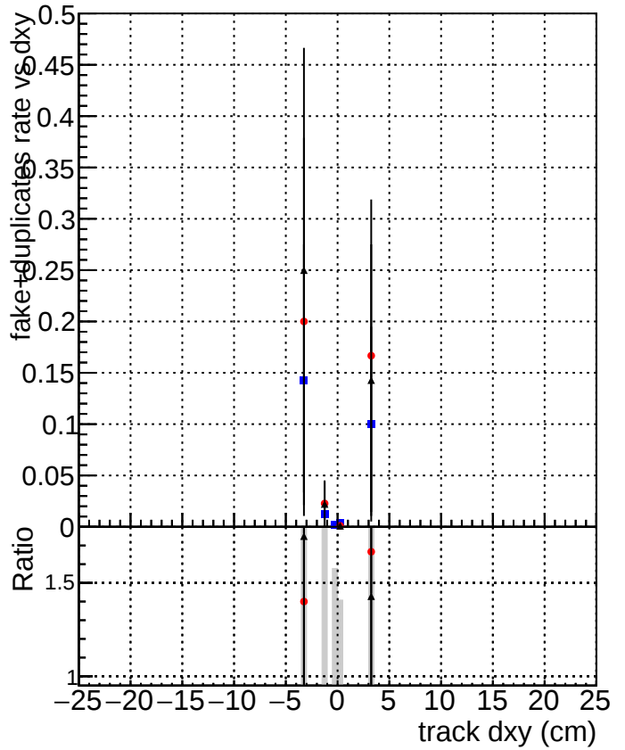
Legend for the plots: DQMstep3_SoftQCD_CKF (Blue squares) DQMstep3_SoftQCD_default (Red circles) DQMstep3_SoftQCD_defaultNEWT3 (Black triangles)
