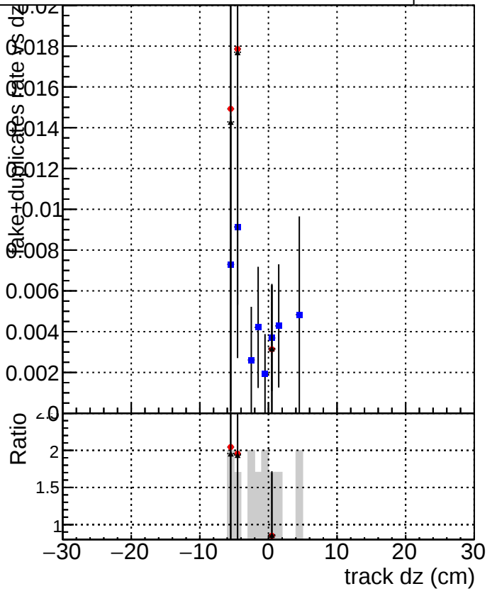
Legend for the plots: DQMstep3_SoftQCD_CKF (Blue squares) DQMstep3_SoftQCD_default (Red circles) DQMstep3_SoftQCD_defaultNEWT3 (Black triangles)
