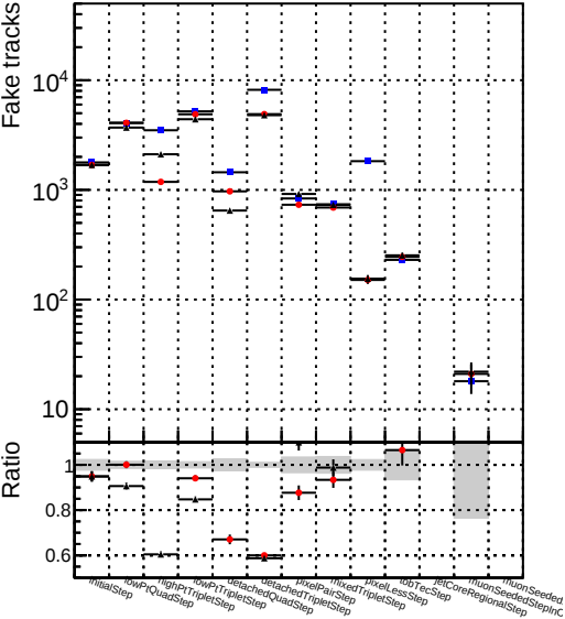
Legend: Blue line: DQMstep3_SoftQCD_CKF Red line: DQMstep3_SoftQCD_default Black line: DQMstep3_SoftQCD_defaultNEWT3
