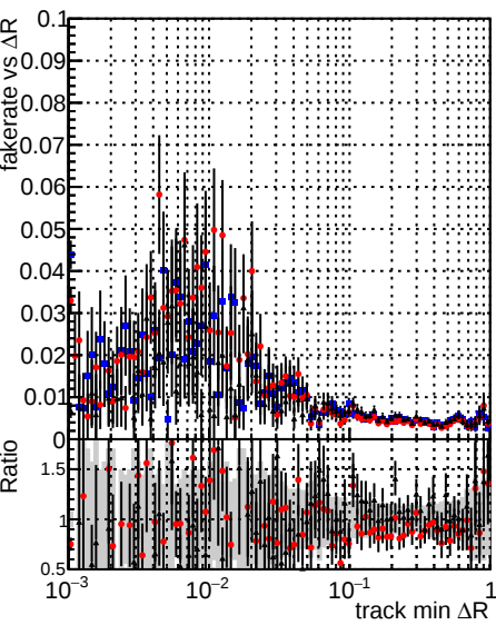
Legend: DQMstep3_SoftQCD_CKF (black), DQMstep3_SoftQCD_default (red), DQMstep3_SoftQCD_defaultNEWT3 (blue)
