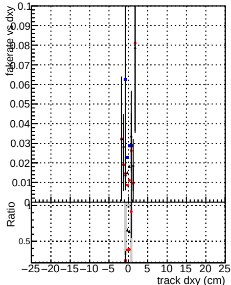
DOMstep3 SoftOCD-CKF DOMstep3 SoftOCD default DOMstep3 SoftOCD default NEWT3
