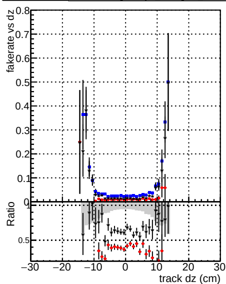
DOMstep3 SoftOCD-CKF DOMstep3 SoftOCD default DOMstep3 SoftOCD default NEWT3
