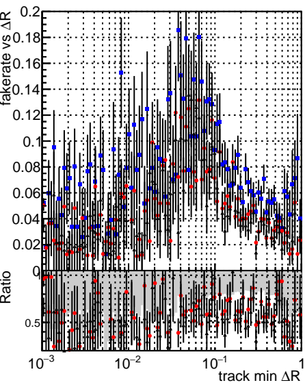
Fake rate vs —●— DQMstep3_SoftQCD_CKF —●— DQMstep3_SoftQCD_default —●— DQMstep3_SoftQCD_NEWT3
