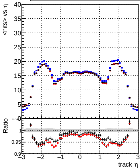
mean hits vs \eta — DQMstep3_SoftQCD_CKF — DQMstep3_SoftQCD_default — DQMstep3_SoftQCD_defaultNEWT3
