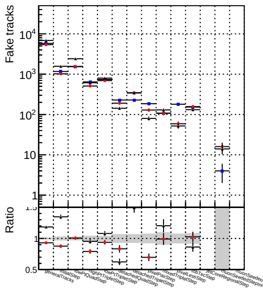
Number Legend 1 DQMstep3_SoftQCD_default 2 DQMstep3_SoftQCD_defaultNEWT3
