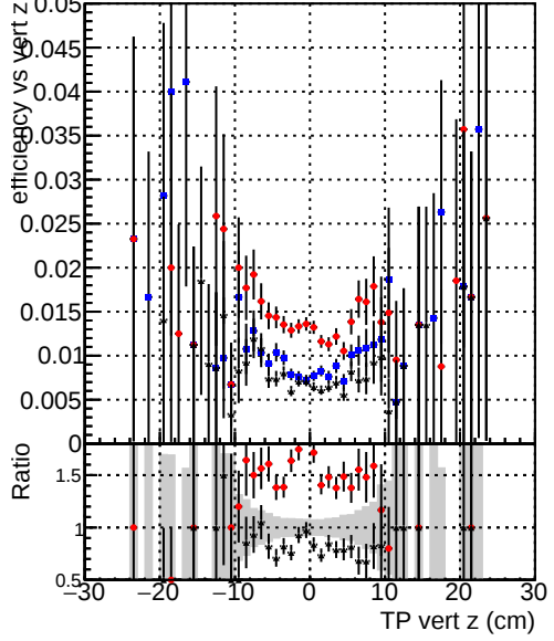
Efficiency vs. TP vert z (cm) — DQMstep3_SoftQCD_CKF — DQMstep3_SoftQCD_default — DQMstep3_SoftQCD_defaultNEWT3
