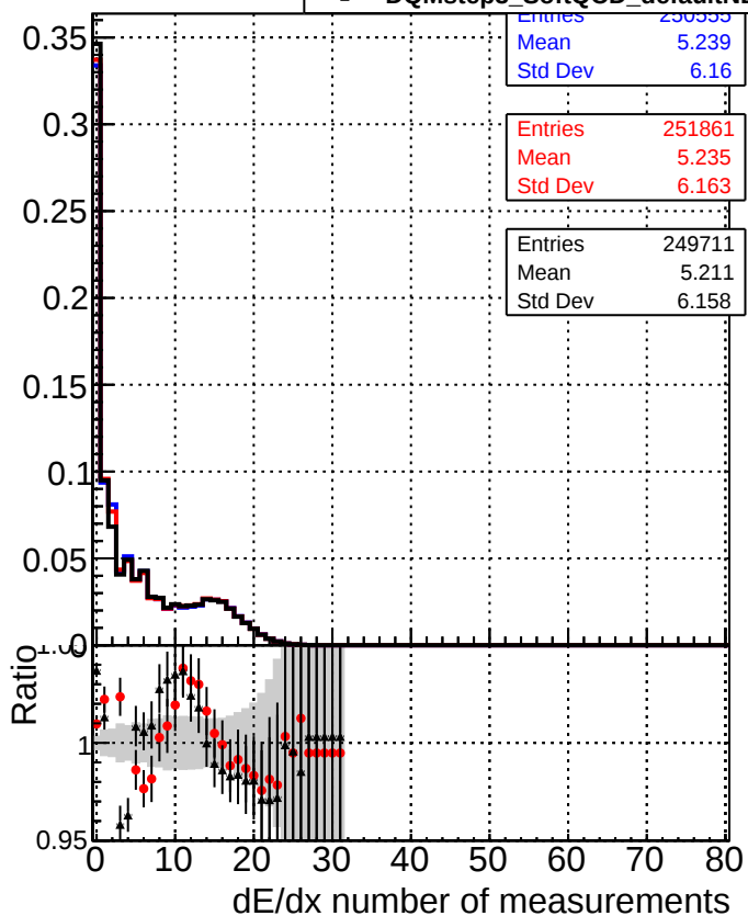
— DQMstep3_SoftQCD_CKF — DQMstep3_SoftQCD_default — DQMstep3_SoftQCD_defaultNEWT3
