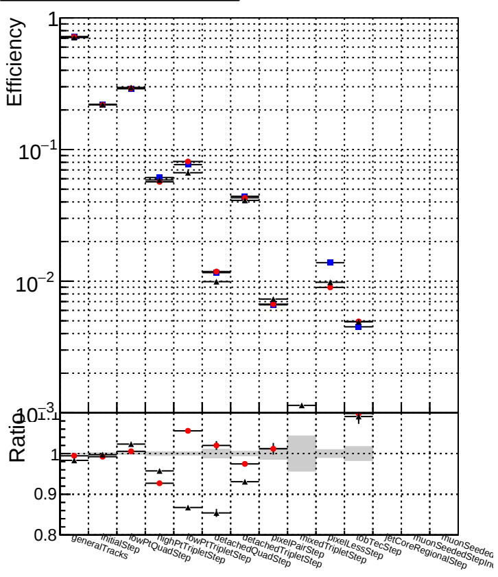
DQMstep3_SoftQCD_CKF DQMstep3_SoftQCD_default DQMstep3_SoftQCD_defaultNEWT20
