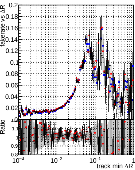
Legend: DOMstep3_SoftQCD_CKF (blue circles) DOMstep3_SoftQCD_default (red circles) DOMstep3_SoftQCD_defaultNEWT20 (black circles)
