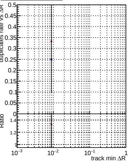
Legend: DQMstep3_SoftQCD_CKF (blue dots), DQMstep3_SoftQCD_default (red dots), DQMstep3_SoftQCD_NEWT20 (black line with error bars)
