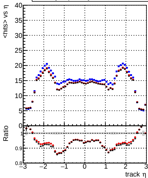
mean hits — DQMstep3_SoftQCD_CKF — DQMstep3_SoftQCD_default — DQMstep3_SoftQCD_defaultNEWT20
