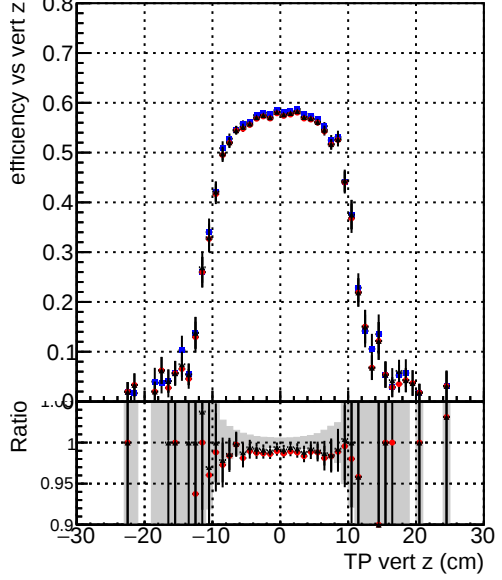
Efficiency vs. sim PV z —●— DQMstep3_SoftQCD_CKF —●— DQMstep3_SoftQCD_default —●— DQMstep3_SoftQCD_defaultNEWT20
