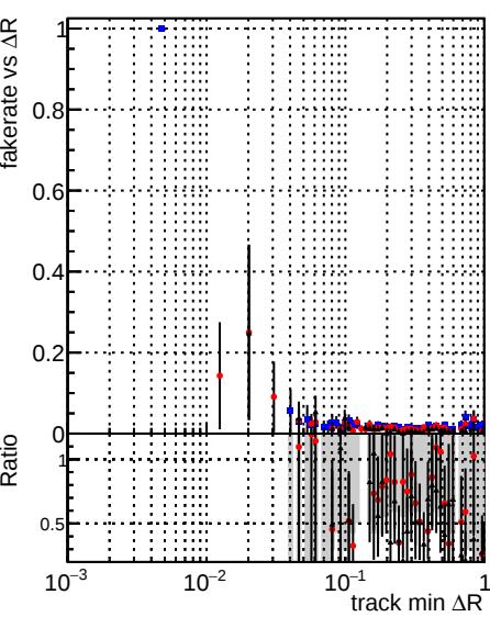
Legend: DQMstep3_SoftQCD_CKF (blue dots), DQMstep3_SoftQCD_default (red dots), DQMstep3_SoftQCD_defaultNEWT20 (black line)
