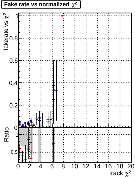
Fake rate vs. DOMstep3 SoftOCD-CKF DOMstep3-SoftOCD-default DOMstep3-SoftOCD-defaultNEW20
