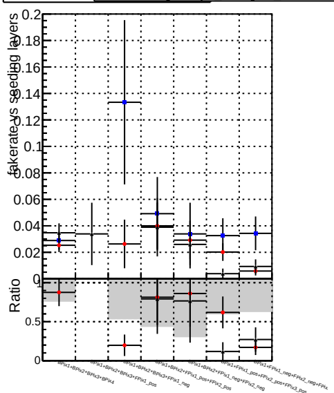
Fake rate vs. DOMstep3 SoftOCD-CKF DOMstep3-SoftOCD-default DOMstep3-SoftOCD-defaultNEW20
