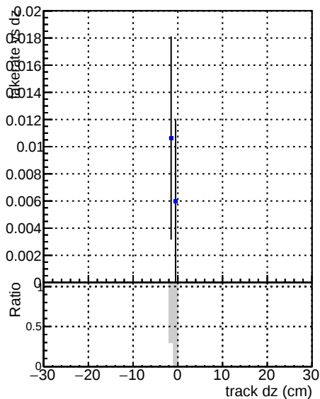
DOMstep3 SoftQCD CKF DOMstep3 SoftQCD default DOMstep3 SoftQCD NEWT20
