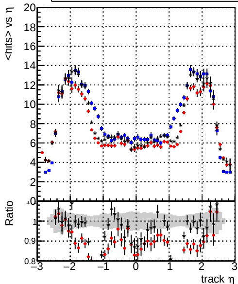
mean hits — DQMstep3_SoftQCD_CKF — DQMstep3_SoftQCD_default — DQMstep3_SoftQCD_defaultNEWT20
