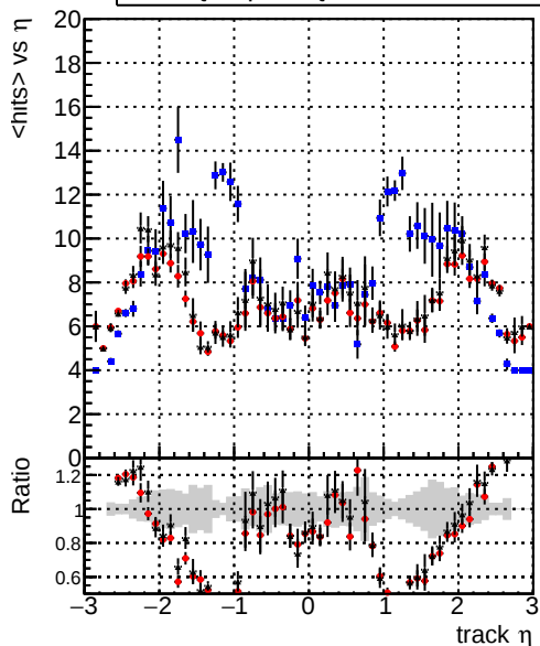
mean hit — DQMstep3_SoftQCD_CKF — DQMstep3_SoftQCD_default — DQMstep3_SoftQCD_defaultNEWT20
