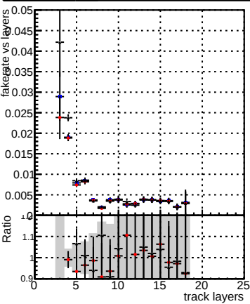
Fake rate vs hit DQMstep3_SoftQCD_CKF DQMstep3_SoftQCD_default DQMstep3_SoftQCD_defaultNEW20
