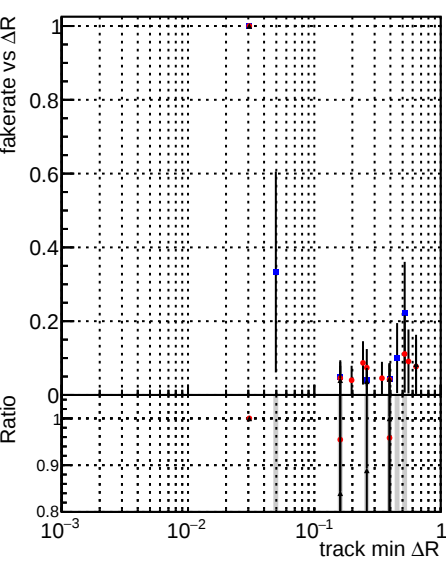
Fake rate vs \Delta R(\text{track}, \text{jet}) DQMstep3_SoftQCD_CKF DQMstep3_SoftQCD_default DQMstep3_SoftQCD_defaultNEWT20
