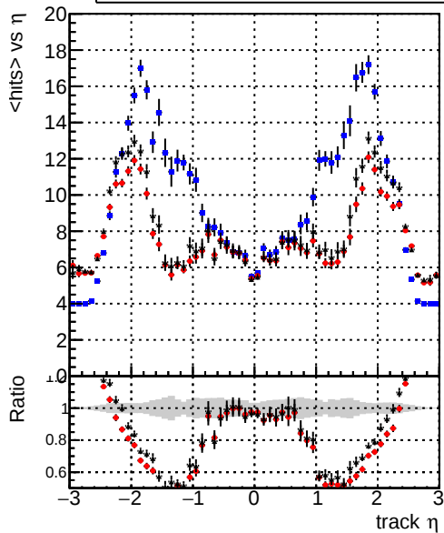
mean hits vs \eta — DQMstep3_SoftQCD_CKF — DQMstep3_SoftQCD_default — DQMstep3_SoftQCD_defaultNEWT20
