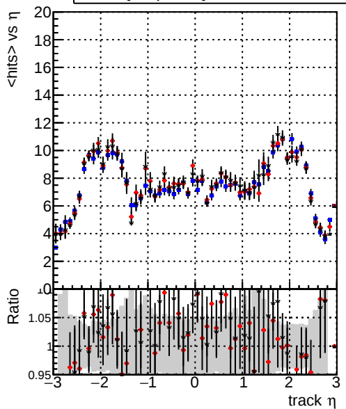
DQMstep3_SoftQCD_CKF DQMstep3_SoftQCD_default DQMstep3_SoftQCD_defaultNEWT20 mean hits
