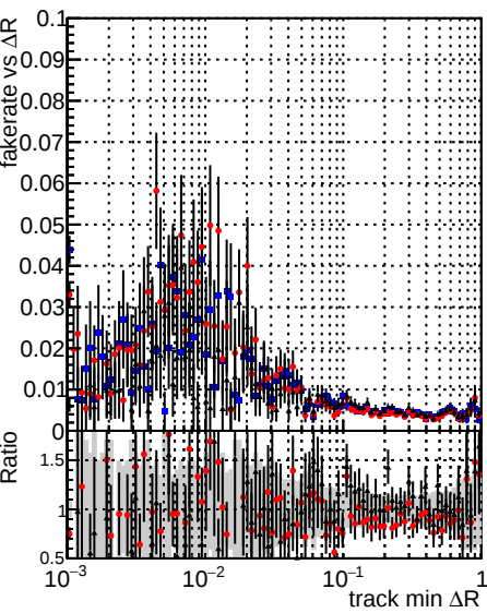
Legend: DQMstep3_SoftQCD_CKF (black), DQMstep3_SoftQCD_default (red), DQMstep3_SoftQCD_defaultNEWT20 (blue)
