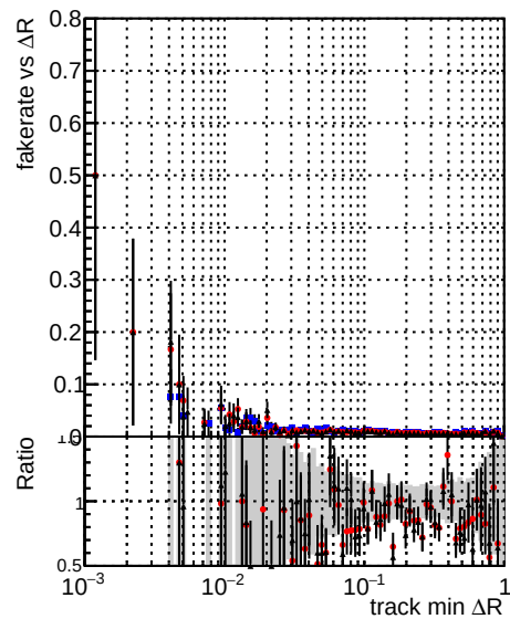
DOMstep3_SoftQCD_CKF DOMstep3_SoftQCD_default DOMstep3_SoftQCD_NEWT20
