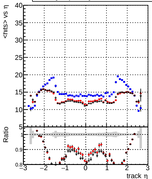
mean hit — DQMstep3_SoftQCD_CKF — DQMstep3_SoftQCD_default — DQMstep3_SoftQCD_defaultNEWT20
