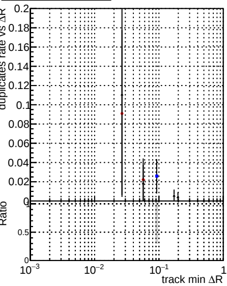
Legend: DQMstep3_SoftQCD_CKF (blue squares), DQMstep3_SoftQCD_default (red circles), DQMstep3_SoftQCD_defaultNEWT20 (black triangles)
