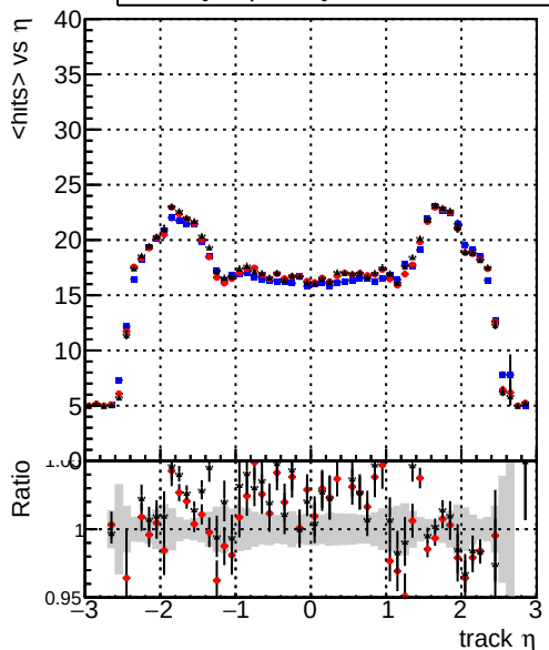
mean hits — DQMstep3_SoftQCD_CKF — DQMstep3_SoftQCD_default — DQMstep3_SoftQCD_defaultNEWT20
