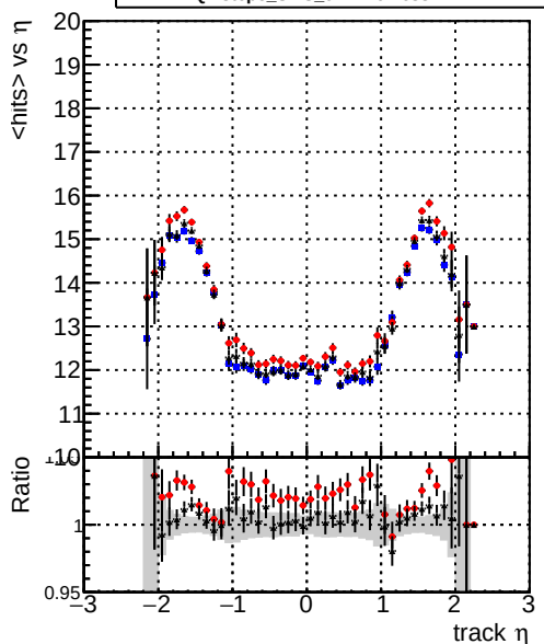
DQMstep3_SMS_CKF DQMstep3_SMS_default DQMstep3_SMS_ckfPixelLess mean hit
