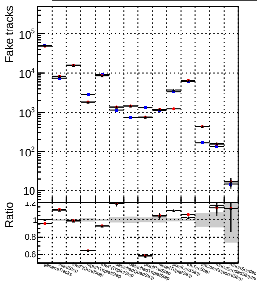
Number Legend 1 DQMstep3_SMS_default 2 DQMstep3_SMS_ckfPixelLess
