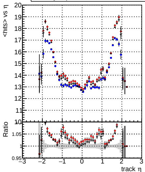
DQMstep3_SMS_CKF DQMstep3_SMS_default DQMstep3_SMS_ckfPixelLess mean hits
