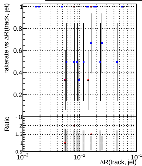
Legend: DQMstep3_SMS_CKF (blue circles) DQMstep3_SMS_default (red circles) DQMstep3_SMS_ckfPixelLess (black circles)
