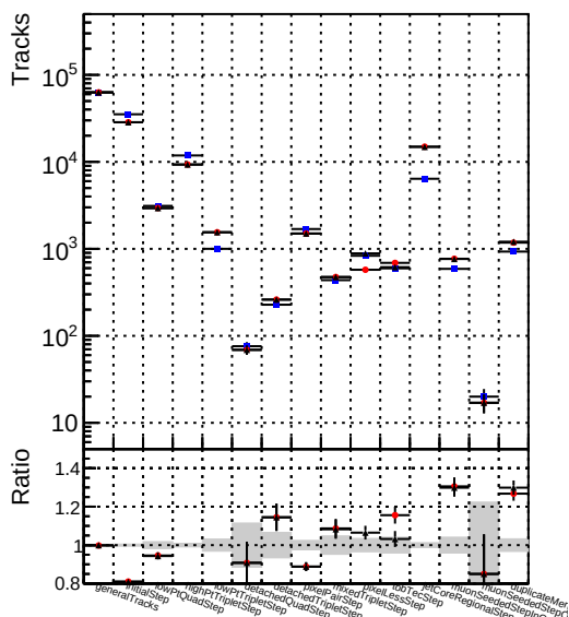
Number of tracks vs collection Legend: DQMstep3 SMS_CKF (blue circles) DQMstep3 SMS_default (red circles) DQMstep3 SMS_ckfPixelLess (black circles)
